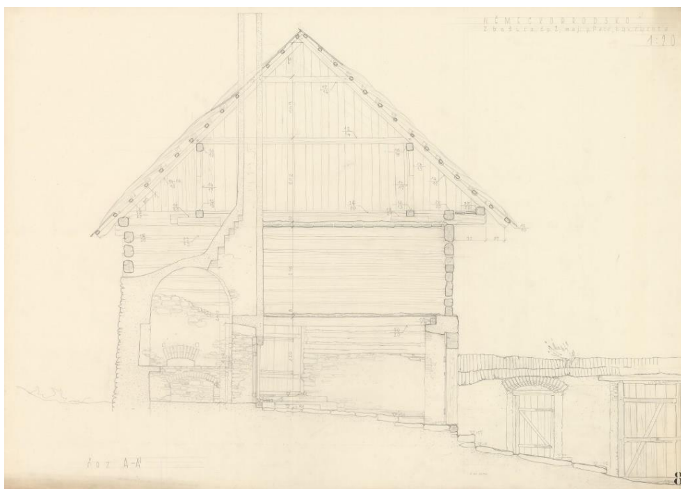
Zbožice, řez černou kuchyní
